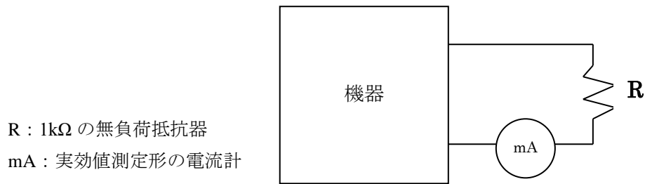
図 A.1 出力電流測定回路
